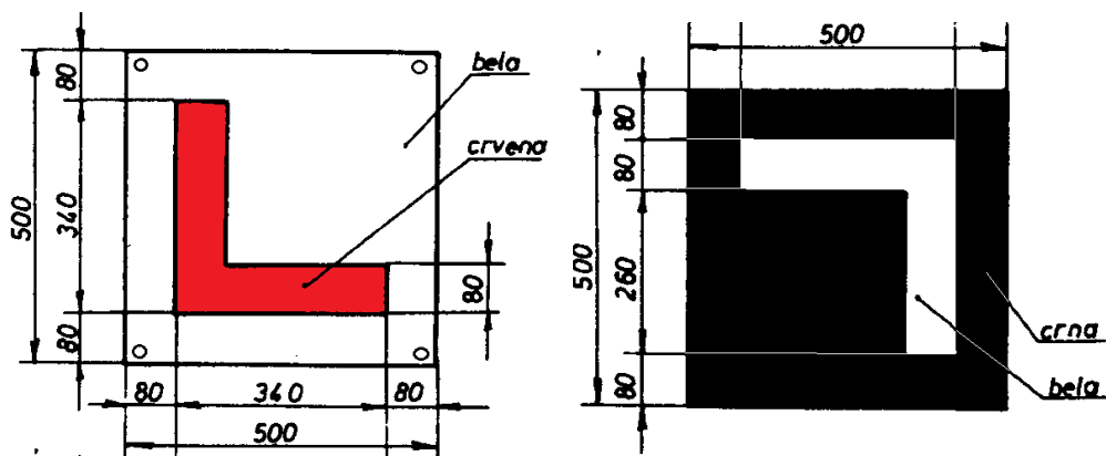
Слика 1. Сигнални знак 216/217 500x500
