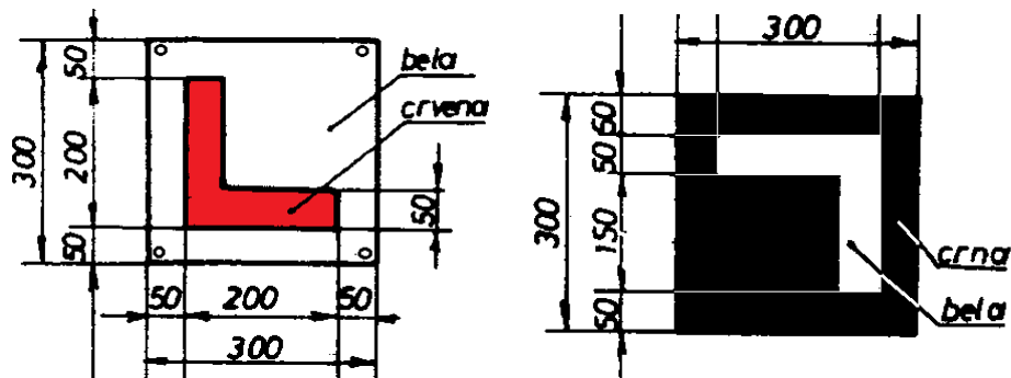
Слика 2. Сигнални знак 216/217 300x300
