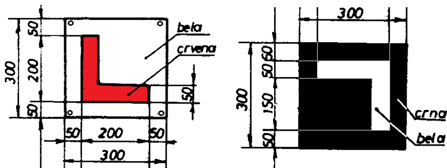
Слика 2. Сигнални знак 216/217 300x300
