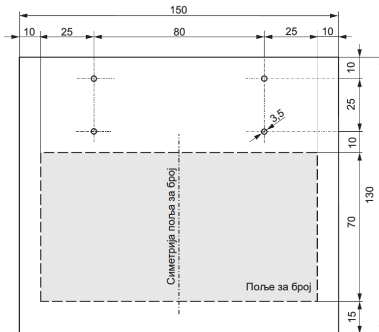
Слика 3. Плочица ознаке
