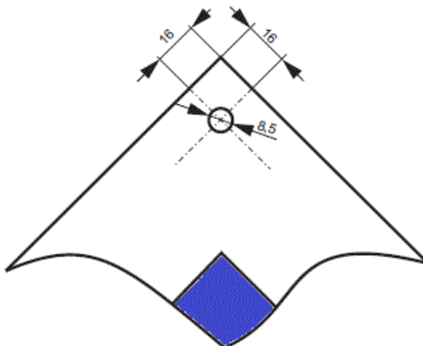
Слика 1. Позиција рупе на сигналном знаку
